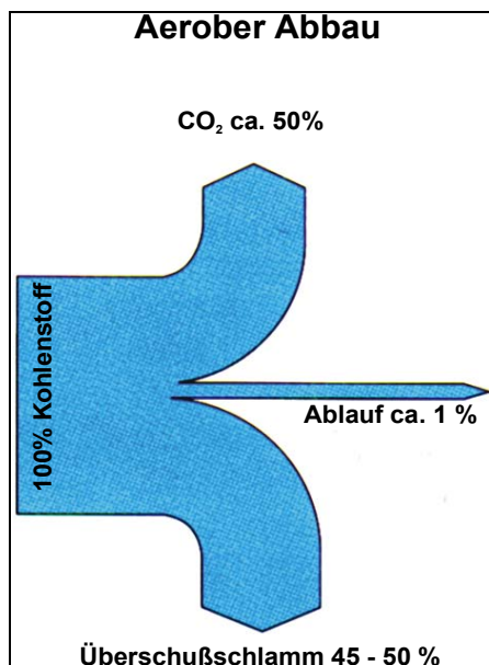
Vergleich der Kohlenstoffbilanz des anaeroben mit dem aeroben mikrobiellen Abbau von Kohlenstoffverbindungen
